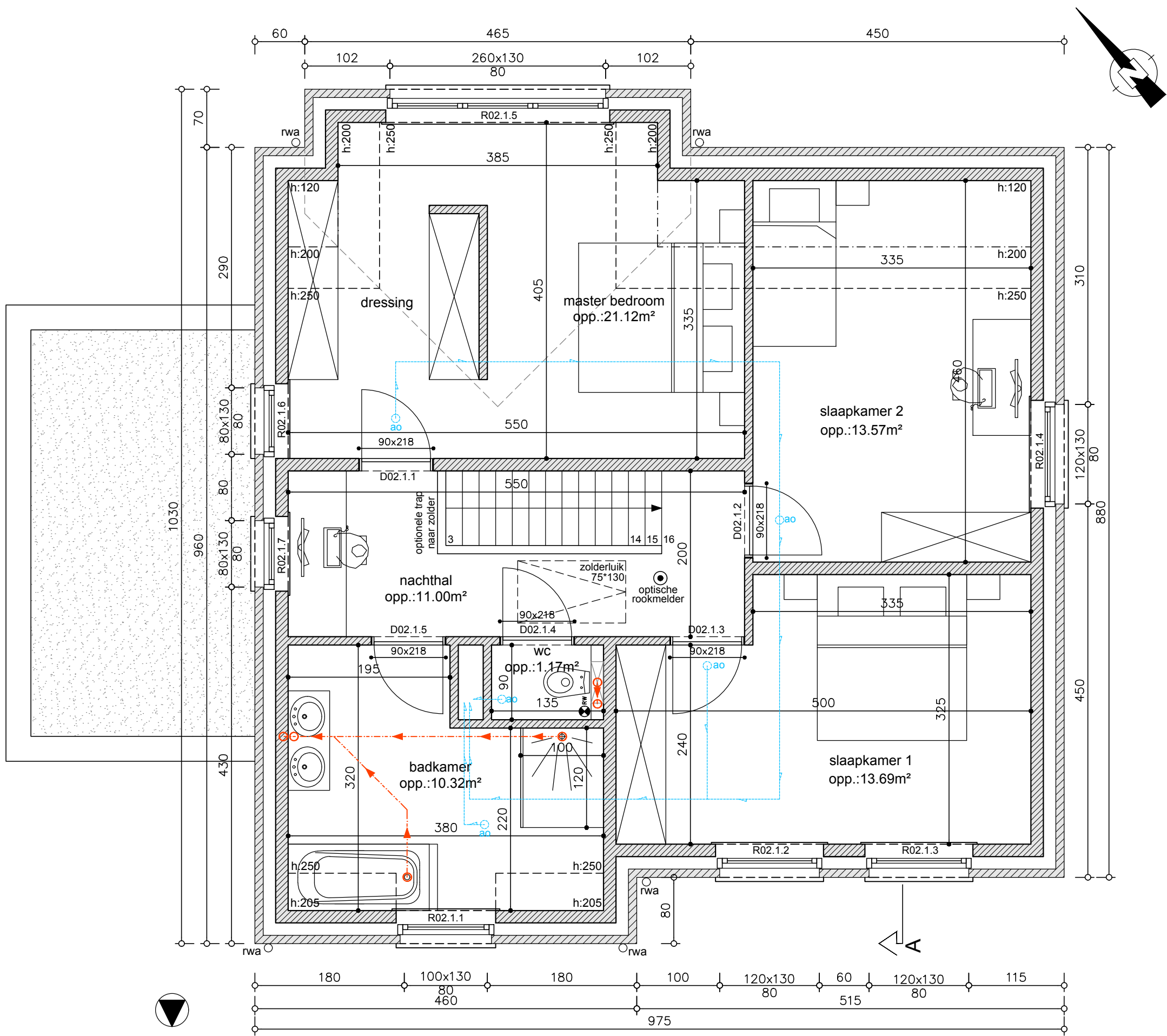
1ste VERDIEPING
